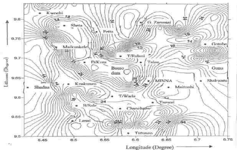
FIG.4 CONTOU MAP OF AQUIFER THICKNESS (CONTOU THICKNESS 2m)
