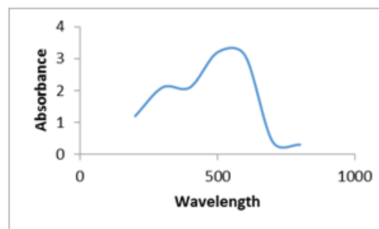
Fig. 2: UV-Visible Spectrum CuNPs (Eucalyptus)
