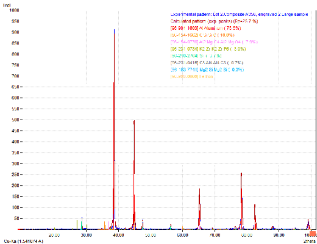
Figure.15. Radiogramme de diffraction X du composite A356
