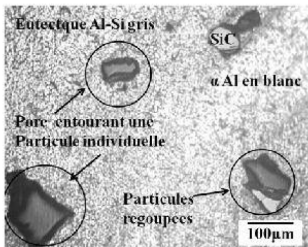
Figure.20. Micrographie optique. Plages pauvres en particules
