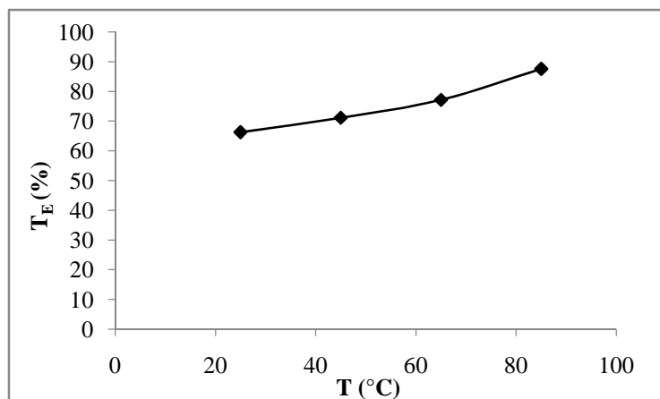
Figure 10. Variation du taux dépuration avec la température ( [\text{H}_2\text{SO}_4]=150 \text{ g.L}^{-1} + [\text{Fe(II)}]=26 \text{ g.L}^{-1} ); Membrane CMX ; 50 \text{ mL.min}^{-1} ; densité: 20 \text{ mA.cm}^{-2} ; 7 h)
