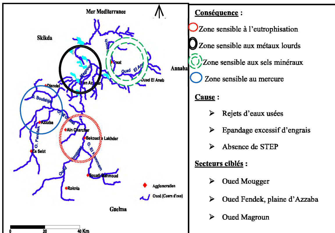
Figure 6. Etat de qualité global des eaux de surface du bassin versant de l'Oued Kebir Ouest.
