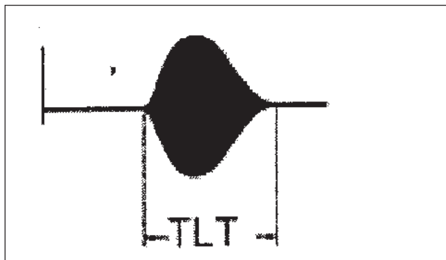
Fig. 6. TEG lysis.
