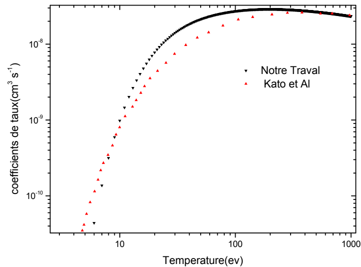
Fig.1. Coefficients de taux d'ionisations pour l'He
