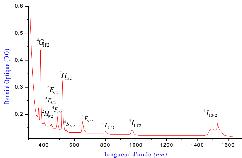
Fig.1. Spectre d'absorption de verre 90NaPO_3-9PbCl_2-1ErF_3
