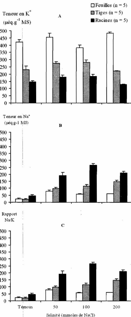
Fig. 2 : A- Teneur en K^+ ( \mu\text{eq/g} MS) des feuilles, tiges et racines en fonction de la concentration du milieu en NaCl (mM). B- Teneur en Na^+ ( \mu\text{eq/g} MS) des feuilles, tiges et racines en fonction de la concentration du milieu en NaCl (mM). C- Variation du rapport Na/K dans feuilles, tiges et racines en fonction de la concentration du milieu en NaCl (mM).
