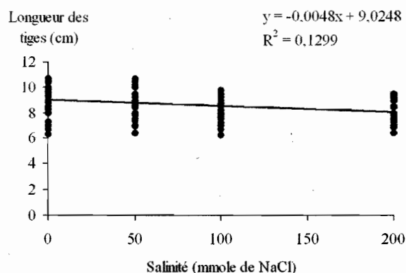
Fig.3 : Evolution de la longueur des tiges (cm) en fonction de la concentration du milieu en NaCl (mM).
