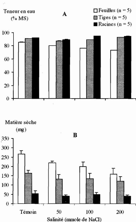
Fig. 1 : A- Teneur en eau (% MS) des feuilles, tiges et racines en fonction de la salinité du milieu (mM NaCl). B- Variation de la matière sèche (mg) des feuilles, tiges et racines en fonction de la salinité du milieu (mM NaCl).
