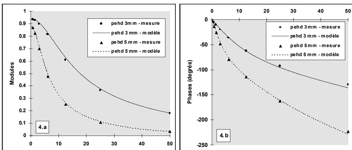
Figure 4: Amortissement de température en fonction de la fréquence de modulation (4.a: Modules - 4.b: Phases)
