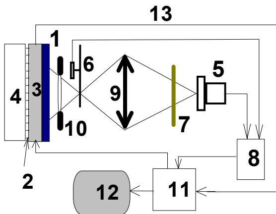
Figure 2: Système de détection infrarouge
