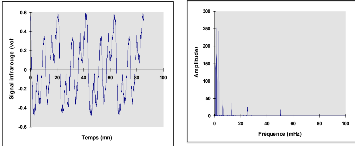
Figure 3: Allure du signal infrarouge mesuré, et le spectre d'amplitude correspondant
