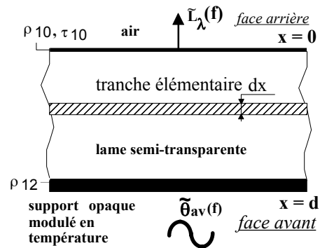
Figure 1 : Lame semi-transparente modulée en température
