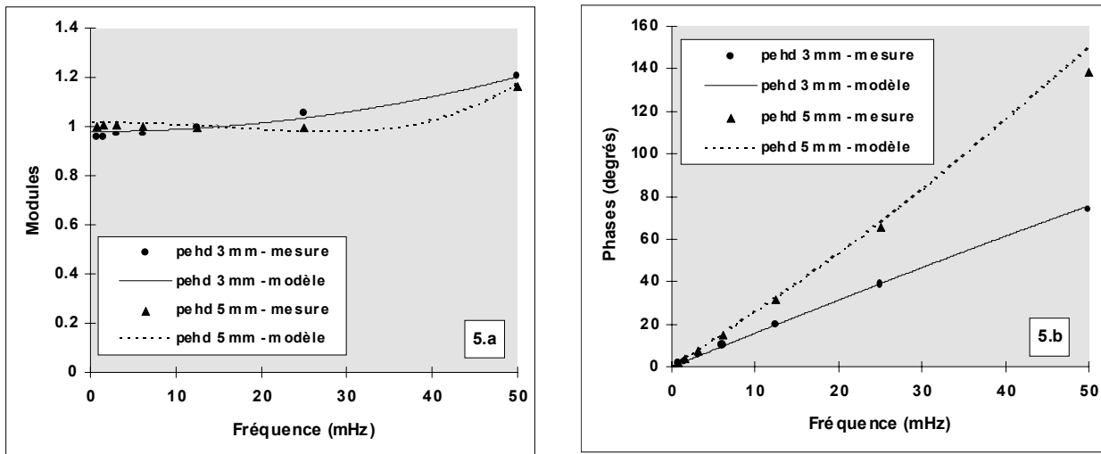
Figure 5: Emissivité apparente des échantillons nus en fonction de la fréquence de modulation (5.a: Modules - 5.b: Phases)
