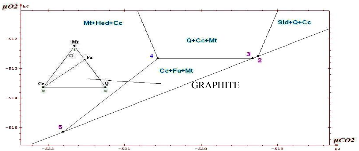
Figure 3b : Suite et détail du champ délimité dans la figure précédente.
