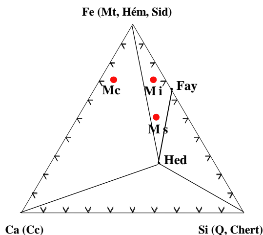
Figure 2 : Compositions moyennes des différents faciès de minerai Mc, Mi, Ms pris en considération dans les calculs thermodynamiques avec les principales phases entrant dans leurs compositions.
