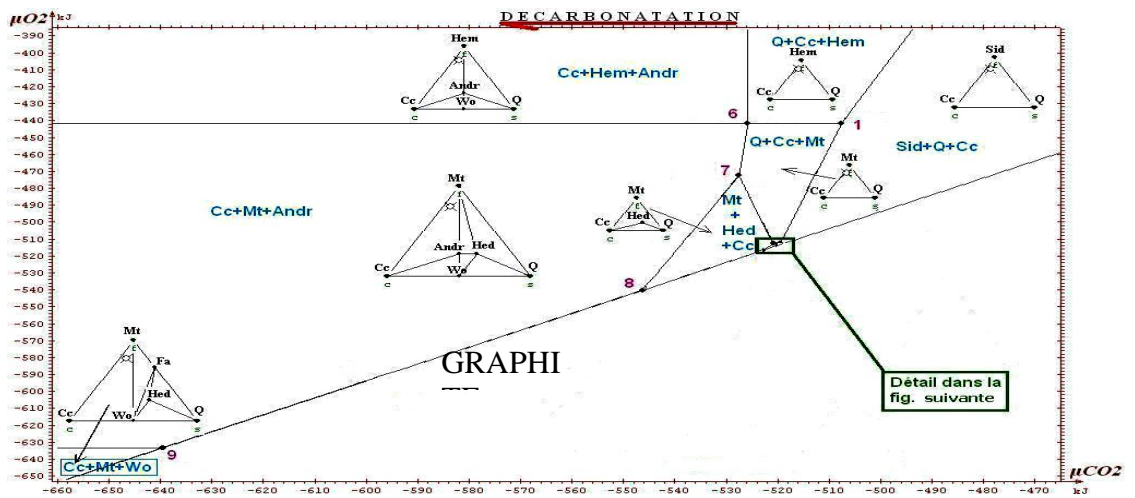
Figure 3a : Diagramme isotherme et isobare (600°C, 6Kb) \mu\text{CO}_2 - \mu\text{O}_2 des phases dans le système Ca-Fe-Si-C-O. Minerai Carbonaté 'Mc'.
