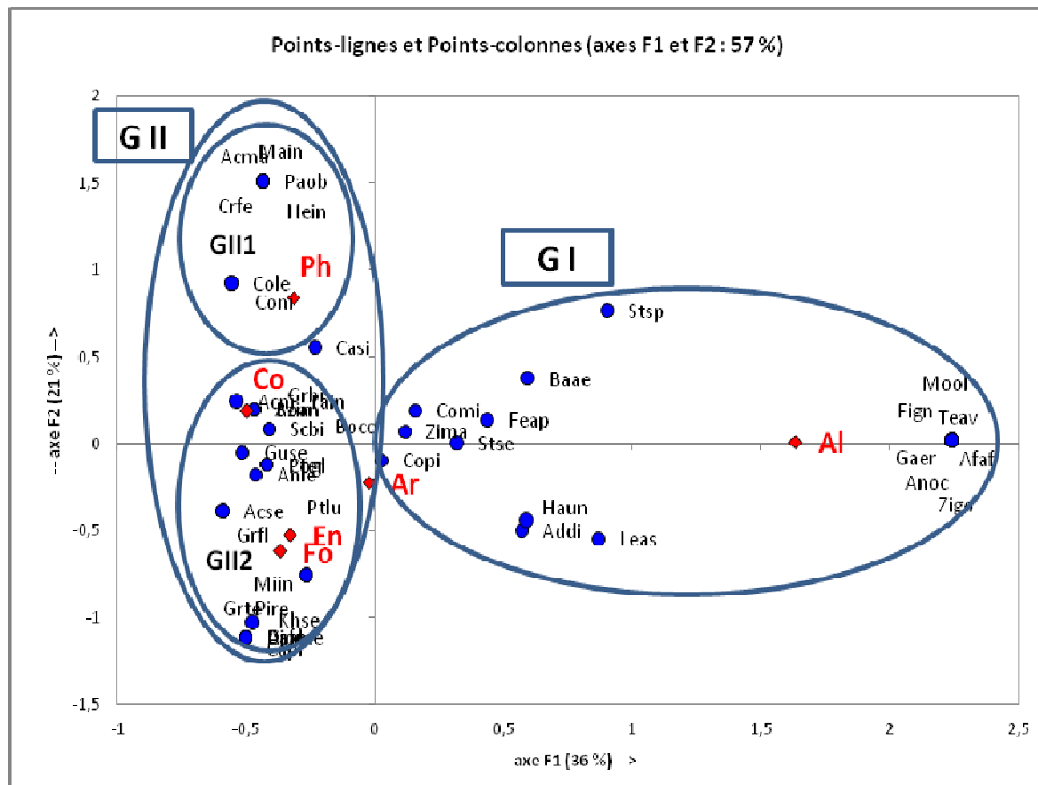
Figure 6 : Projection des individus (espèces) et variables (Usages) sur les plans factoriels F1x2.
